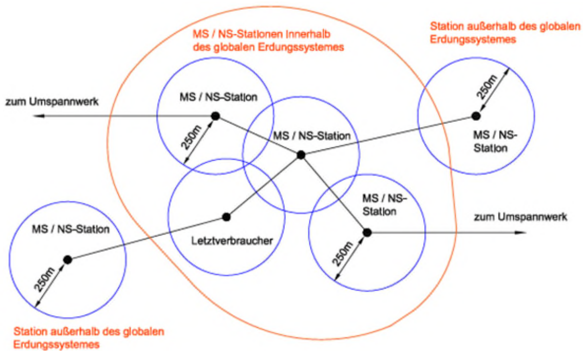
Abb. 1 Globales Erdungssystem
